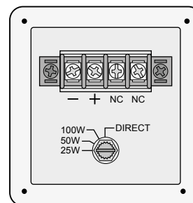
Beispiel PAB-6WP/WS: eingestellte Nennbelastung = 25W Example PAB-6WP/WS: rated load adjusted = 25W
