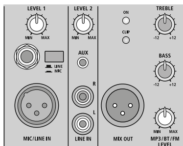
② PAK-8DMP/10DMP Branchements, réglages
