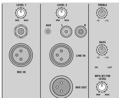
③ PAK-12DMP Anschlüsse, Regler
