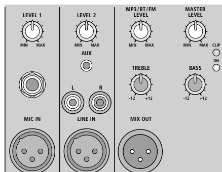
④ PAK-15DMP Collegamenti, regolatori
