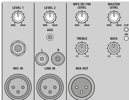
④ PAK-15DMP Conexiones, controles
