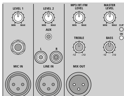
④ PAK-15DMP Branchements, réglages
