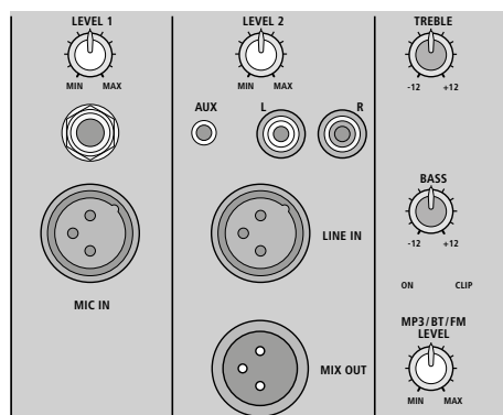
③ PAK-12DMP Branchements, réglages
