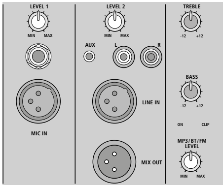
③ PAK-12DMP Conexiones, controles
