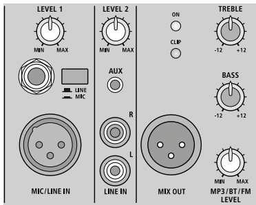
② PAK-8DMP/10DMP Conexiones, controles
