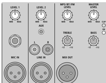
④ PAK-15DMP Anschlüsse, Regler
